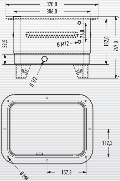
12 LİTRE KAYNAKSIZ KARE TANKI (YAĞ TANKI SETİ)
